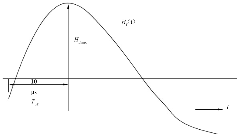
图 F.3 首次雷击磁场强度(10/350 μs)上升期的模拟
